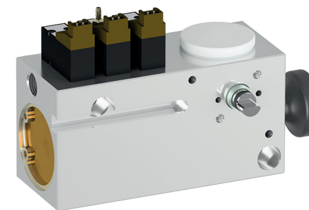
Pneumatischer Drehantrieb mit integrierten Magnetventilen
